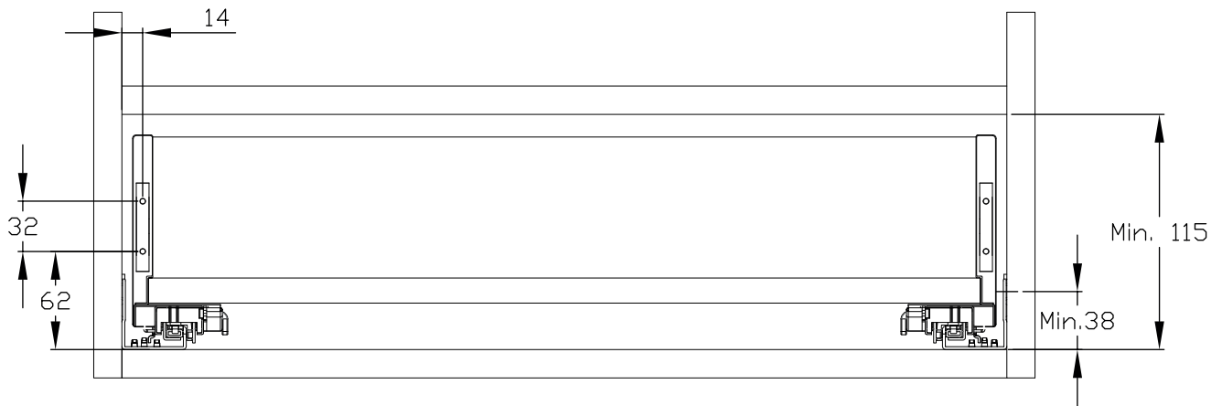
Snello H90
