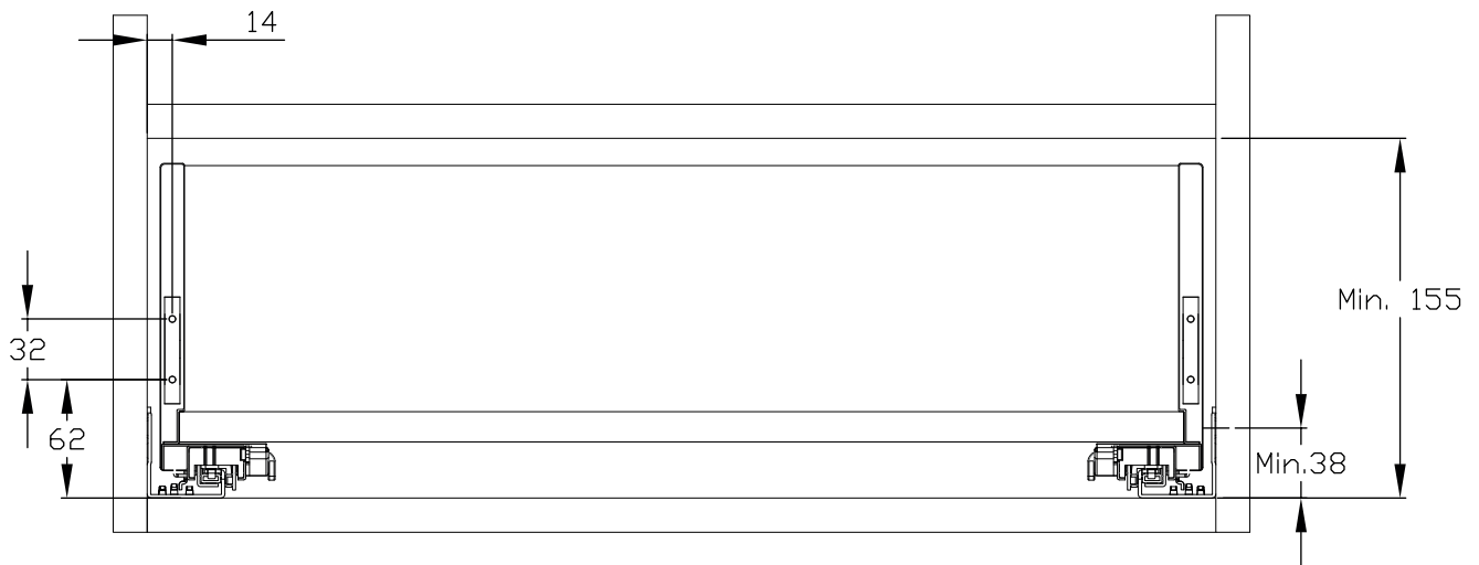
Snello H130
