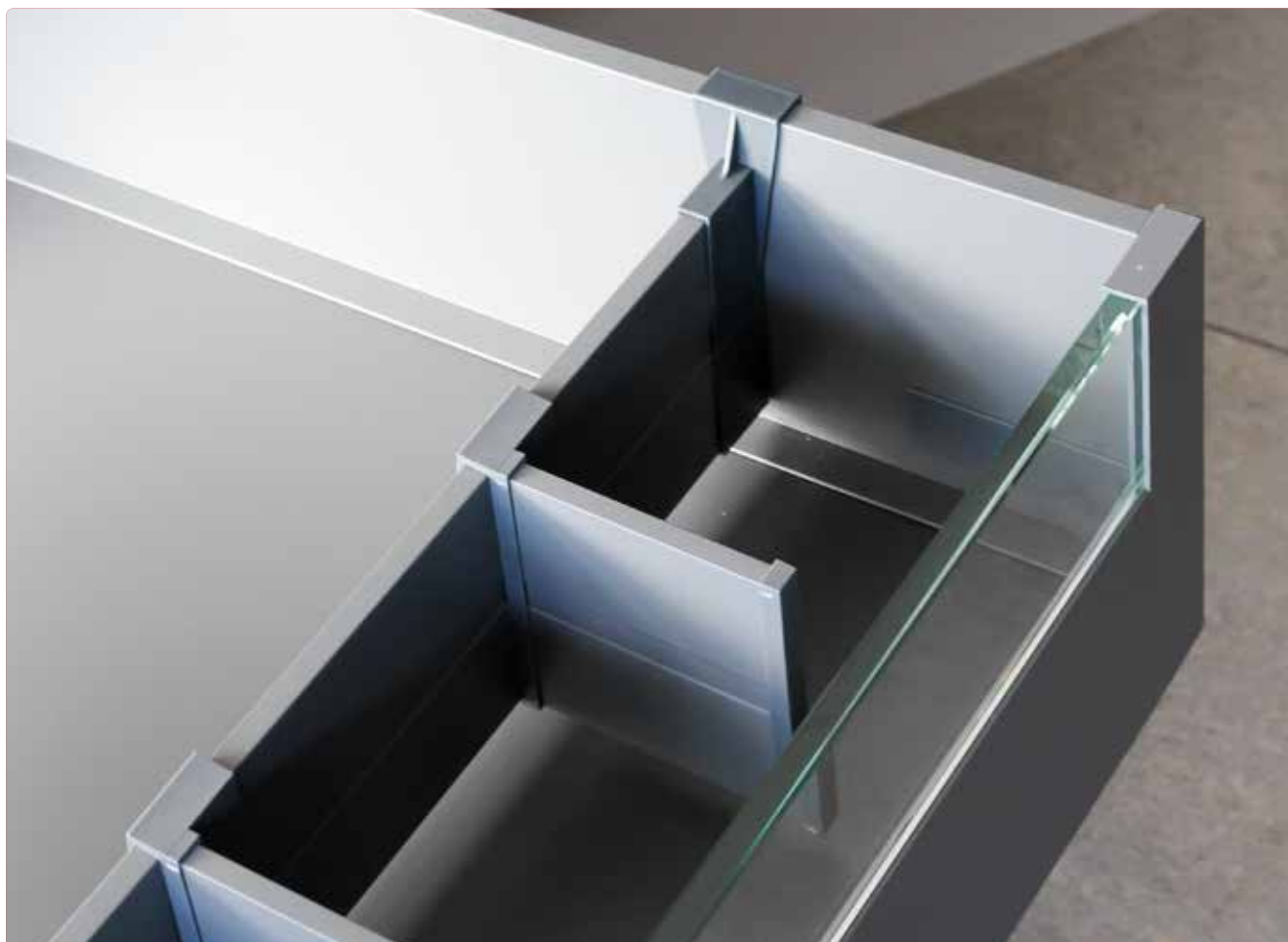
Set fijación lateral + Perfil separador interior Advanced
