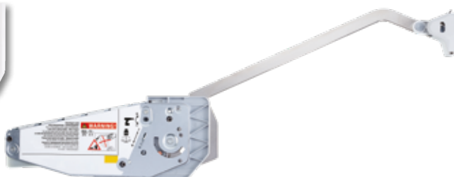
Mecanismo FREEfold
