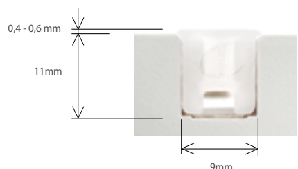
ENCASTRE PLANO
