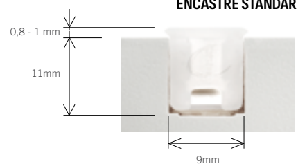
ENCASTRE STANDAR
