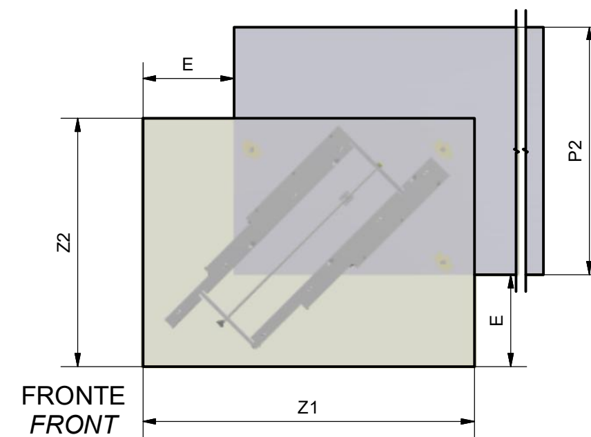
411/78.1243.22 VISTA DALL'ALTO / TOP VIEW
