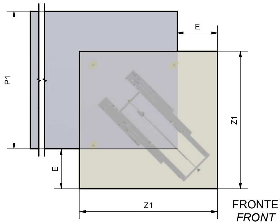
411/78.1241.22 VISTA DALL'ALTO / TOP VIEW
