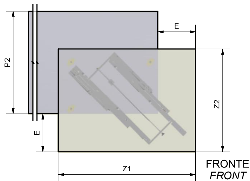
411/78.1242.22 VISTA DALL'ALTO / TOP VIEW
