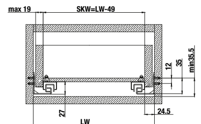
Cajón estandar Standar drawer
