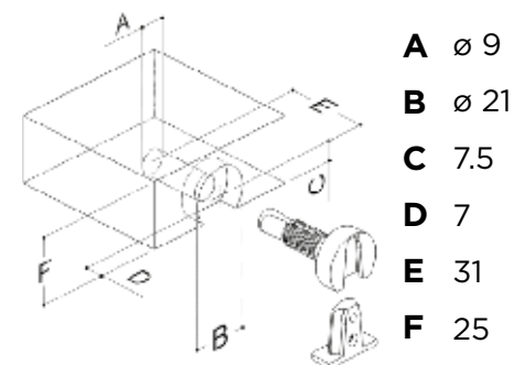
Mecanización bulón
