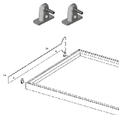
Kit Aluminio soporte externo
