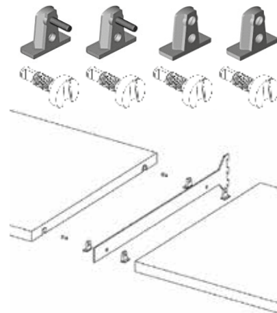
Kit Aluminio soporte central
