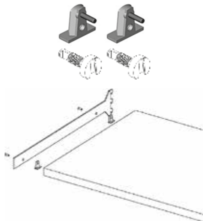
Kit Madera soporte externo
