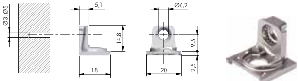
Soporte balda - costado (atornillar)
