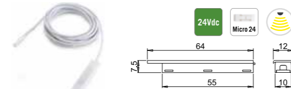
Sensor Nexus superficie IFR
