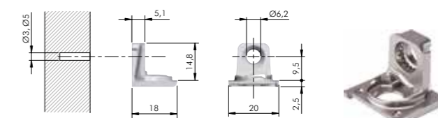
Soporte balda - costado (atornillar)
