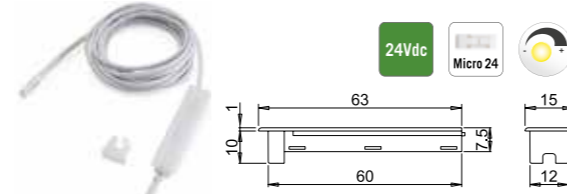
Sensor Nexus encastre Touch SD
