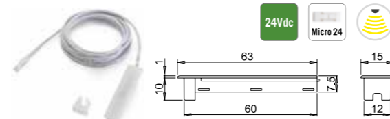
Sensor Nexus encastre IFR
