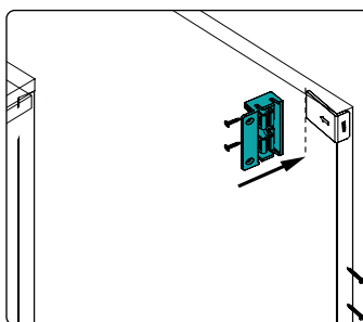
Ejemplo de montaje gola Zero vertical lateral.
