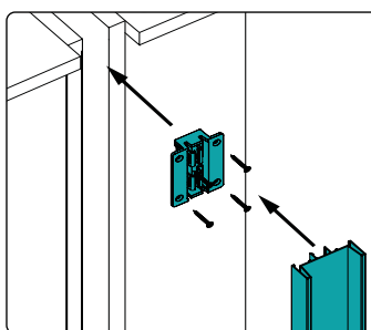
Ejemplo de montaje gola Zero vertical central.
