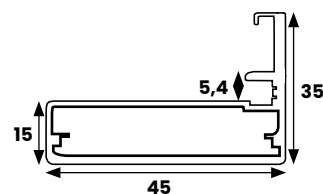
Perfl tirador (TIR)
