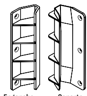
Enganche Soporte Set espaciador trasero (2 enganches + 2 soportes + 12 tornillos)
