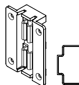
Set fijación gola Zero vertical central (4 fijación + 1 tapa + 16 tornillos)
