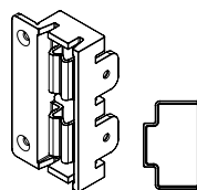
Set fijación gola Zero vertical lateral (4 fijación + 1 tapa + 16 tornillos)
