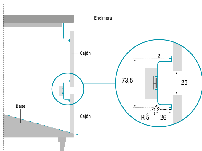
Fijación Metálica Eco
