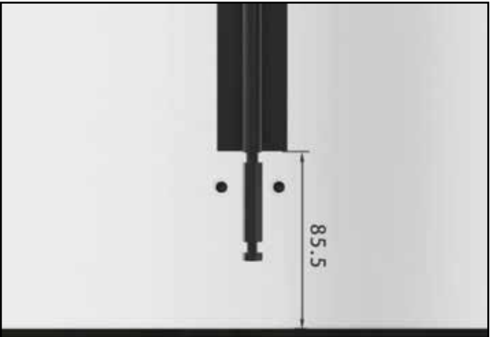
Medida recomendada de corte de perfil cobertor tensor (parte superior / parte inferior), al extremo de la puerta.
