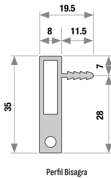
Perfil Bisagra
