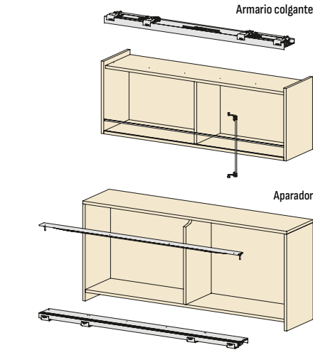
Armario colgante
