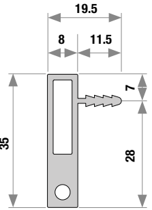
Perfil Tirador
