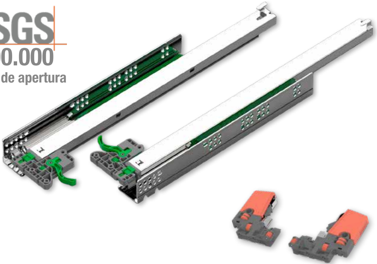
Set manetas guía Variax 3D (OPCIONAL)
