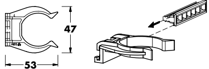
Abrazadera Único
