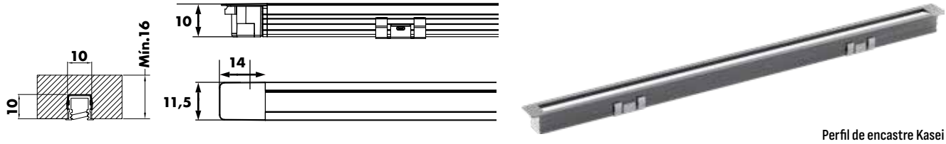
Perfil de encastre Kasei
