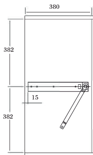
Plano de instalación del riel guía superior
